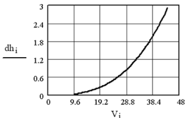
Рисунок 5 – Залежність висоти вітрового нагону dh , м від швидкості вітру V , м/с
