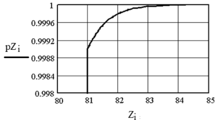
Рисунок 3 – Імовірнісна крива розподілу статичного рівня води перед греблею із ґрунтових матеріалів Z , м Кременчуцького гідровузла
