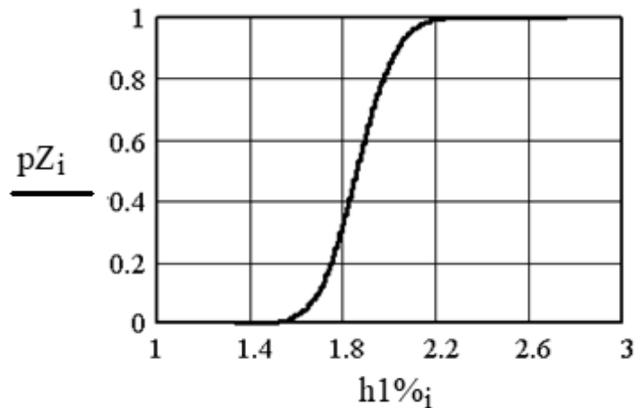
Рисунок 7 – Залежність хвилі 1 % забезпеченості у системі хвиль h_{1\%} , м від випадкової величини – позначки статичного рівня води Z , м
