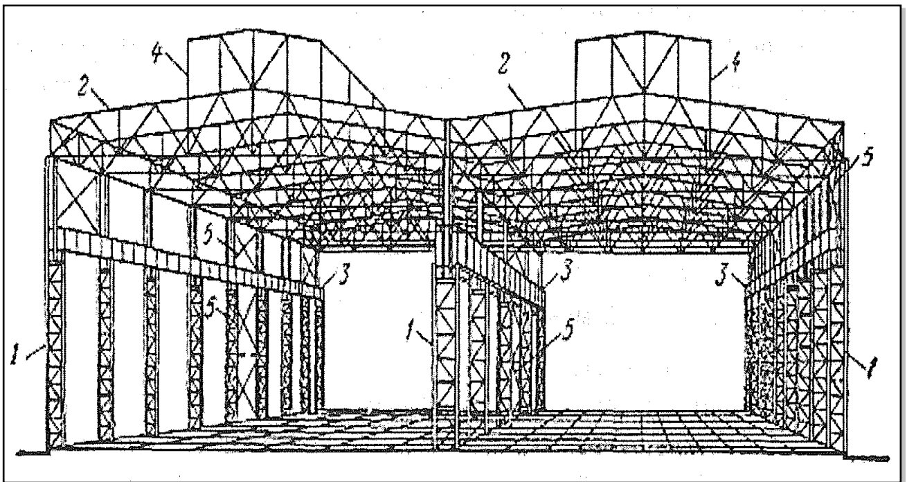
Рисунок 1.1 – Конструктивна схема каркасу двопролітної виробничої будівлі:
