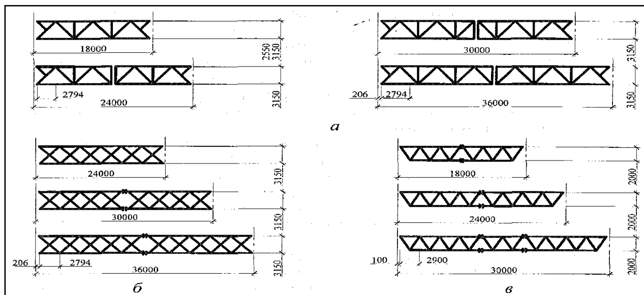
Рисунок 3.5 – Схеми типових ферм з паралельними поясами:
