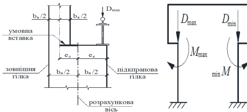
Рисунок 5.11 – Розрахункова схема рами при вертикальних кранових навантаженнях у випадку дії D_{\max} на ліву колонну
