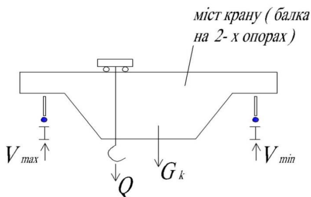
Рисунок 5.8 – Максимальний тиск на ліві колеса мосту крана, до яких найближче розташовується візок з вантажем
