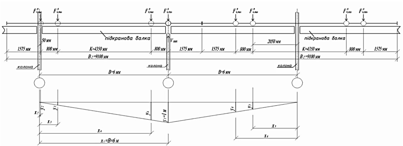
Рисунок 5.9 – Схема розташування коліс зближених кранів на підкранових балках для визначення D_{\max} на колоні
