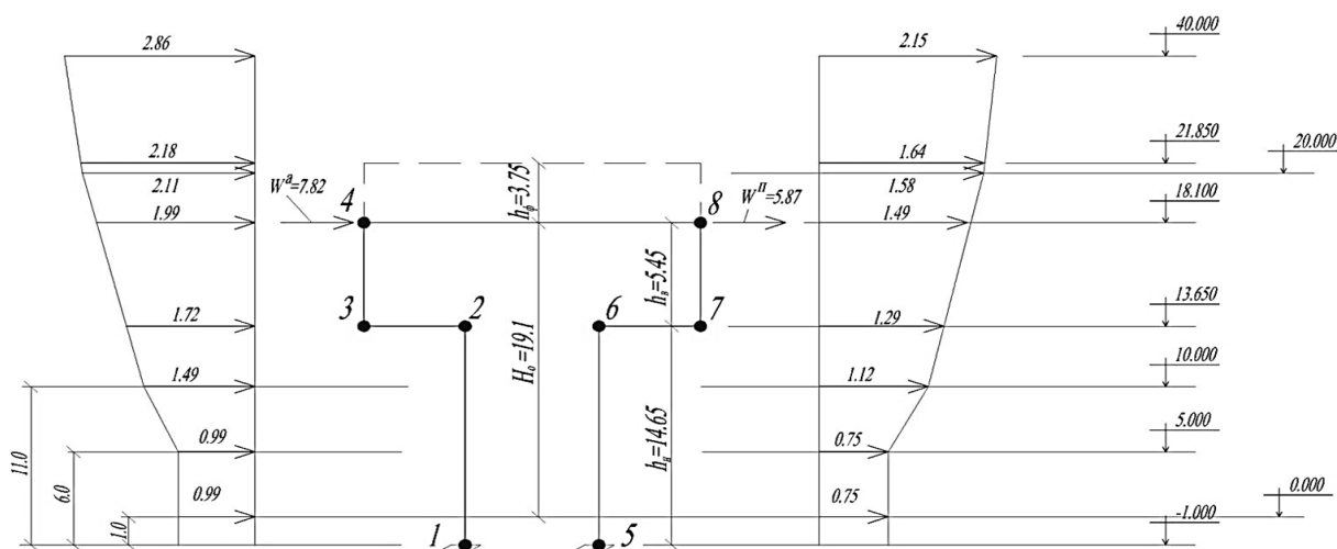
Рисунок 5.15 – Епюри вітрового тиску на поперечну раму
