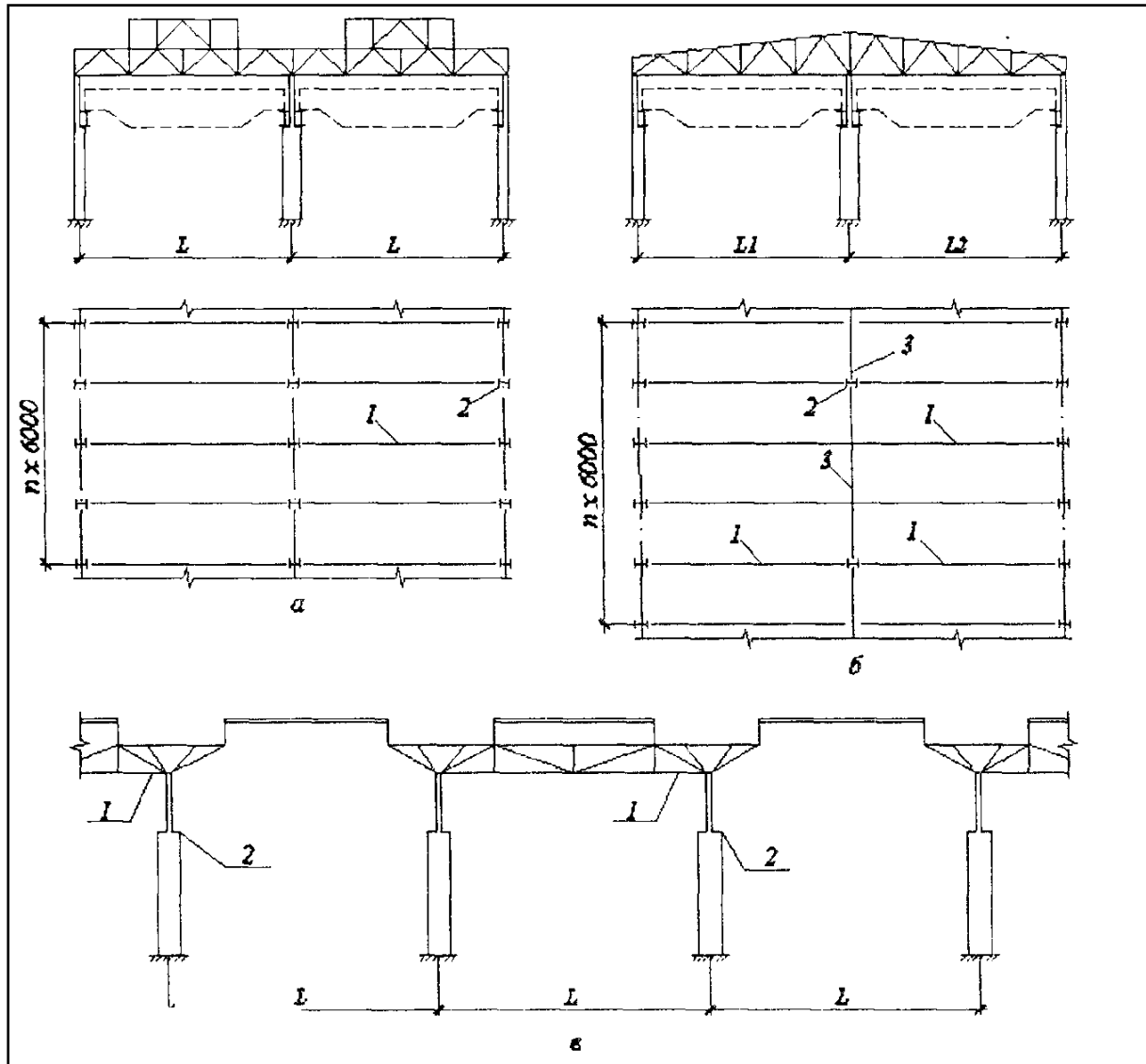
Рисунок 2.2 – Конструктивні схеми багатопролітних каркасів: а – крок колон по зовнішніх і внутрішніх рядах однаковий; б – крок колон по зовнішніх і внутрішніх рядах різний; в – рама з консольними фермами; 1 – кроквяні ферми; 2 – колони; 3 – підкраново-підкроквяна ферма
