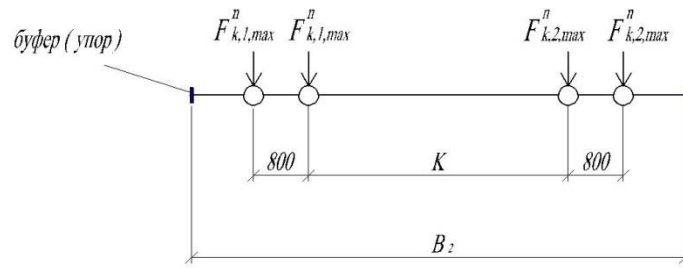
Рисунок 5.7 – Схема крана
