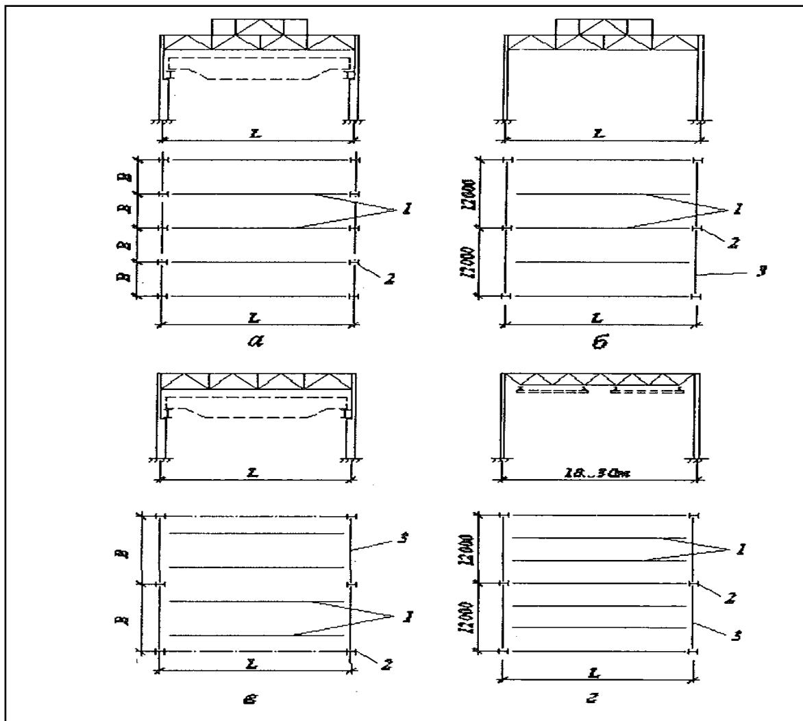
Рисунок 2.1 – Конструктивні схеми однопролітних каркасів: а – крок колон дорівнює кроку ферм; б, в, г – крок колон більший за крок ферм; 1 – кроквяні ферми; 2 – колони; 3 – підкроквяні ферми
