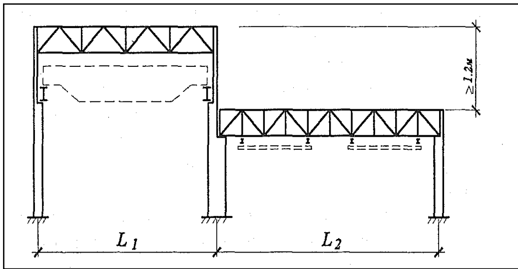
Рисунок 2.3 – Схема рами з прогонами різної висоти і довжини
