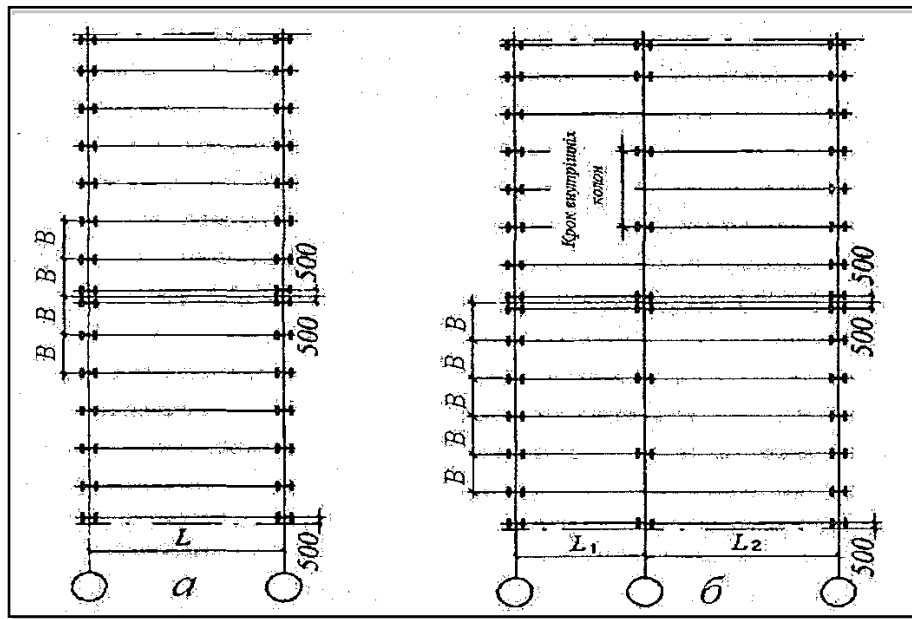
Рисунок 3.3 – Схеми розміщення колон у будівлях: а – однопролітних; б – багатопролітних
