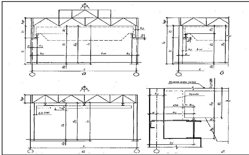
Рисунок 3.4 – До компоновання поперечних рам: а, б – з мостовими опорними кранами; в – з підвісними опорними кранами; г – визначення розмірів при проході збоку
