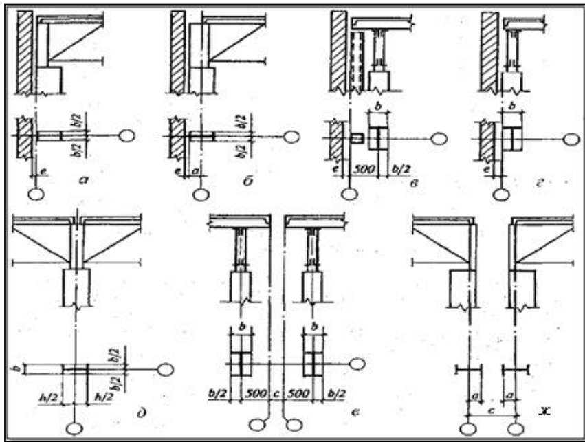
Рисунок 3.2 – Прив’язки колон до координаційних осей: а, б – крайніх рядів; в, г – в торці будівлі; д – середніх рядів; е – поперечних температурних швів; ж – у місцях розташування поздовжніх температурних швів
