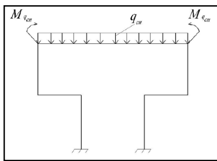
Рисунок 5.6 – Розрахункова схема поперечної рами для снігового навантаження
