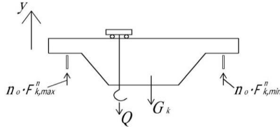
Рисунок 5.10 – Визначення мінімального тиску на колесо крана
