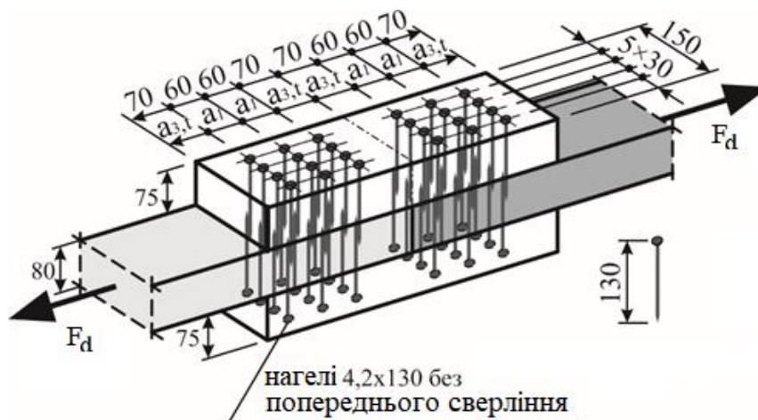
Рисунок 1 – Однозрізне з'єднання деревини з деревиною без попередньо свердлених отворів
