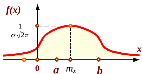
Рисунок 7.5 – Щільність розподілу f(x) Рисунок 7.6 – Інтегральна функція F(x)
