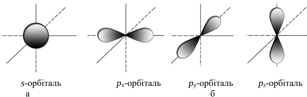
Рисунок 2.1 – Зображення атомних орбіталей: а – s -орбіталь; б – p -орбіталь
